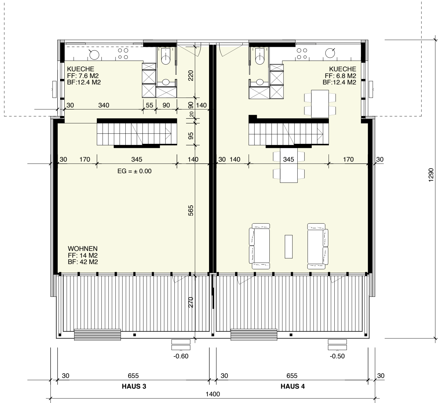
GRUNDRISS ERDGESCHOSS 1 : 100
