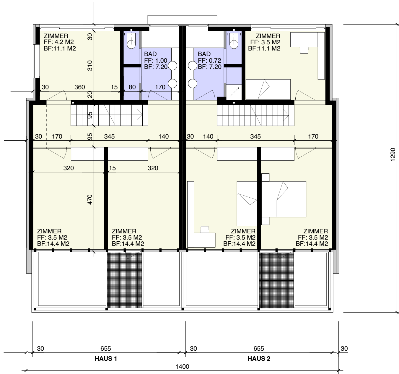
GRUNDRISS OBERGESCHOSS 1 : 100
