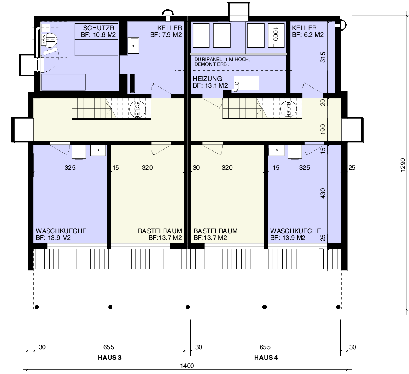
GRUNDRISS UNTERGESCHOSS 1 : 100
